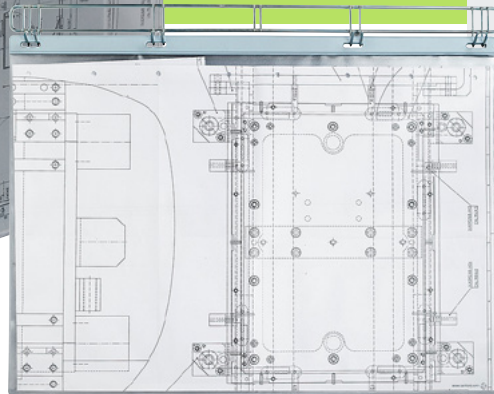
TRaverse FÜR WANDSYSTEM (Befestigung an der Wand)
